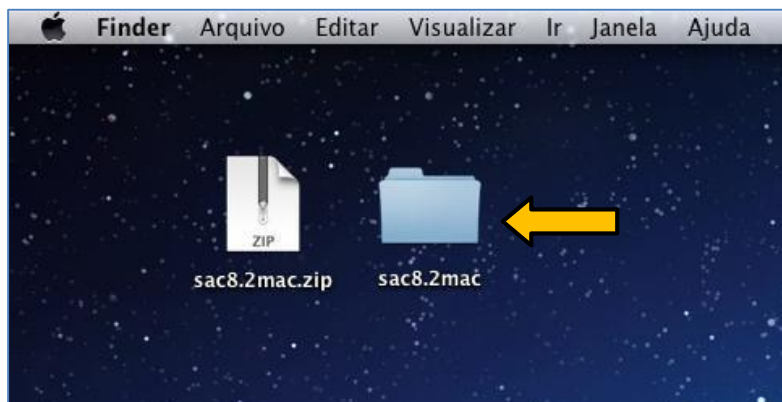
Figura 2 - Pasta Descompactada
