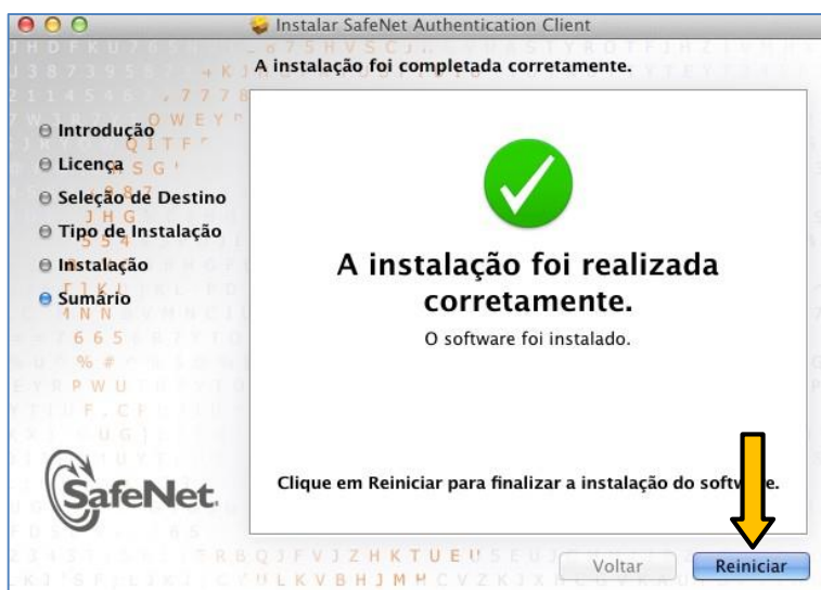
Figura 11 - Instalação OK
